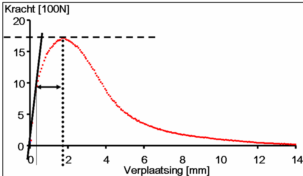
Figuur 4: Voorbeeld resultaat indirecte trekproef
